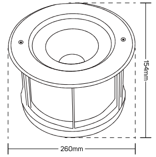
612165 (Cutting Size Ø235)
