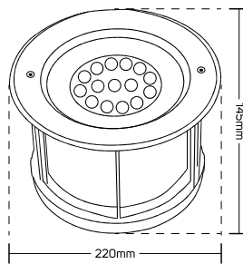
612170 (Cutting Size Ø195)
