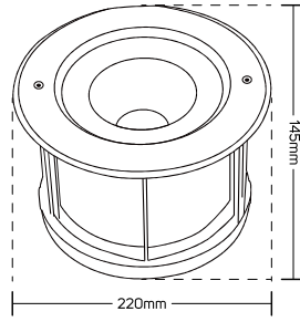
612164 (Cutting Size Ø195)
