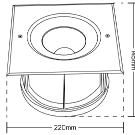
612167 (Cutting Size Ø195)
