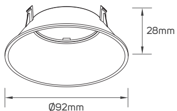
● 613115 - ● 613116 - ● 613117 - Reflector
